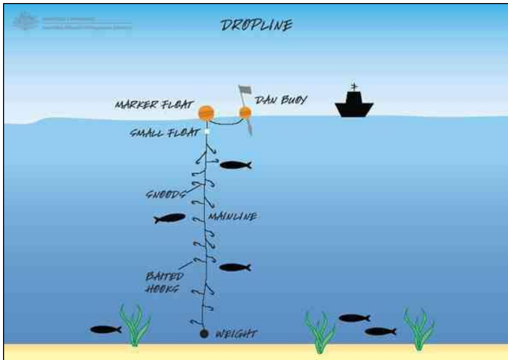
( الشكل ١٠- ٧) السنارة الثابتة ذات الخيط الطويل
