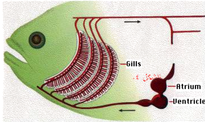
الشكل ٤.٥ جهاز الدوران المغلق في الأسماك
