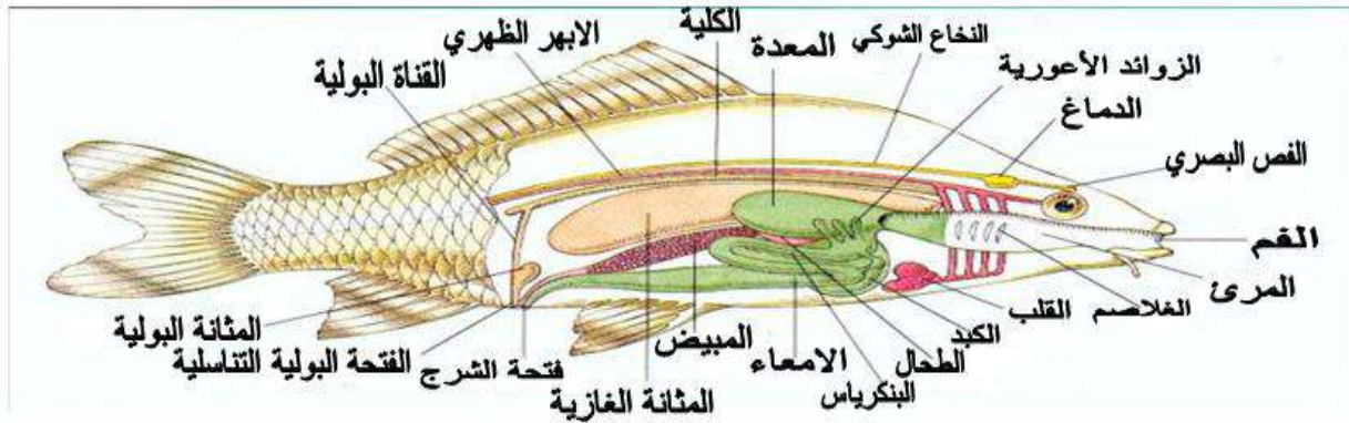
الشكل ٤-١ التشريح الداخلي والجهاز الهضمي في الأسماك
